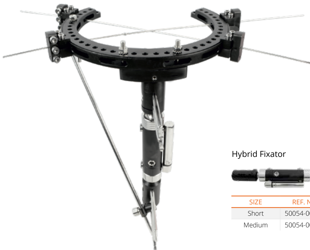
Hybrid Fixator Rod Clamp
